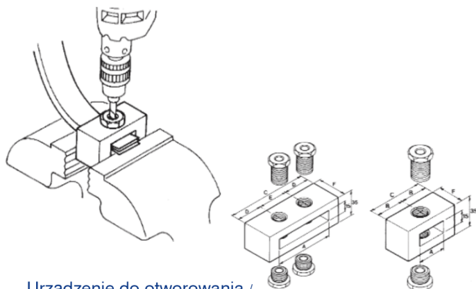
Urządzenie do otworowania / Drilling devices
