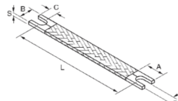
Złącze widelkowe F / Fork terminal F
