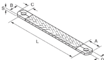
Złącze zaokrąglone T / Curved terminal T
