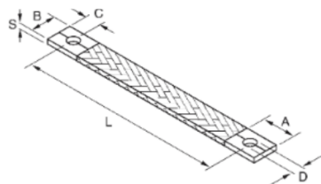
Złącze standardowe D / Standard terminal D
