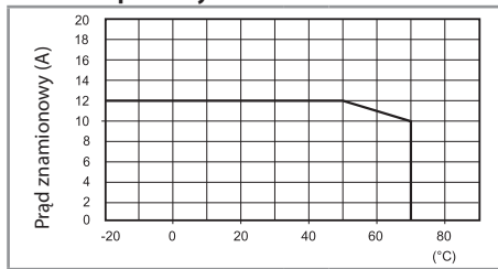
L 96 - Prąd znamionowy względem temperatury otoczenia
